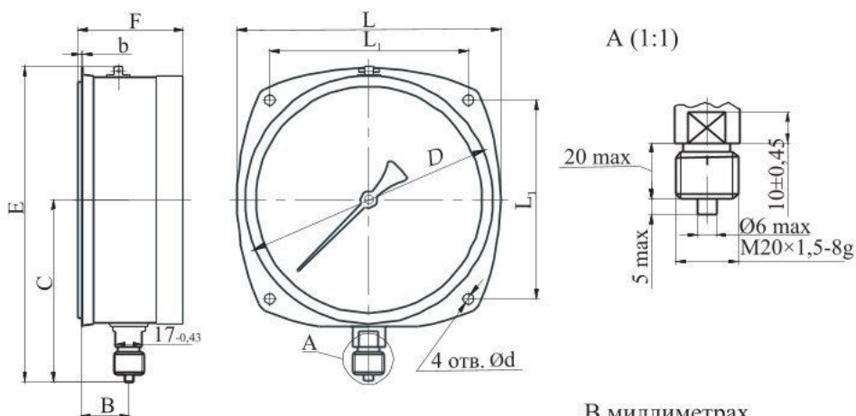
Рисунок 3 - Габаритные и присоединительные размеры приборов
